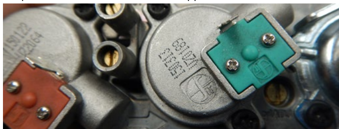
Figure 13.h Réglage des orifices de refoulement
