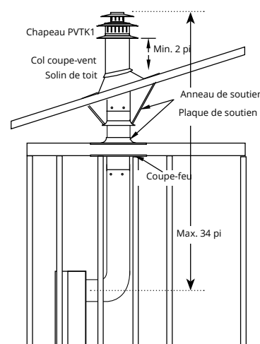
Figure 6.d Ventilation arrière, ventilation montée sur le toit (1 = coude à 90°).
